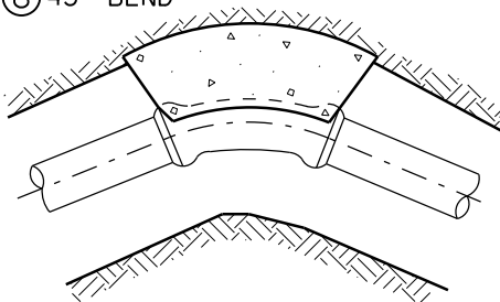
⑧ 45° BEND
