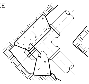
⑧ 45° BEND
