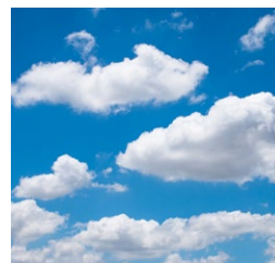
Cumulus
