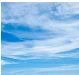
Cirrus
